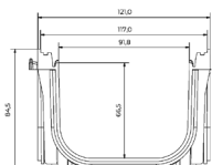
Caniveau polypropylène à fentes avec couvercles PP A15 SCANIV114D
