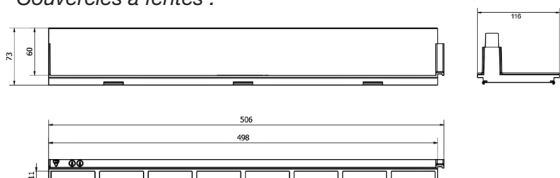
Couvercles à fentes :
