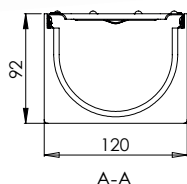
Caniveau polypropylène avec grille en acier galvanisé SCANIV1009
