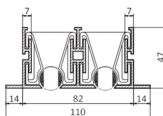
SEZIONE modello a 2 feritoie
