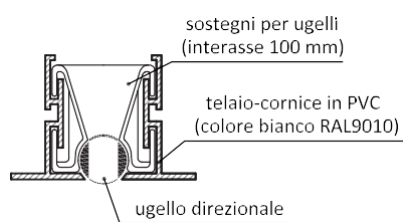
SEZIONE descrittiva
