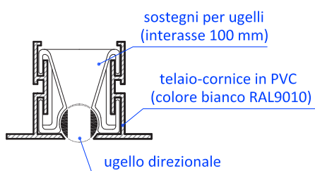
SEZIONE descrittiva
