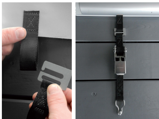
Système d'attache rapide (option)
