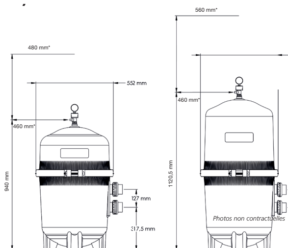
Filtres à cartouches Flow 39 et Flow 49
