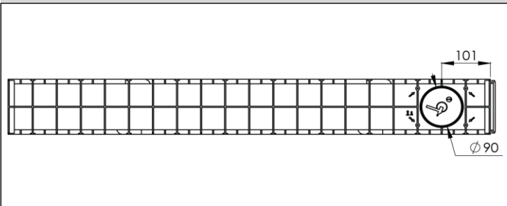
Grille en composite polyamide fentes 6mm
