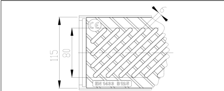
Détails de la grille
