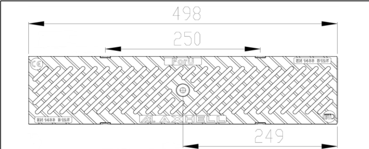
Grille en composite polyamide fentes 6mm
