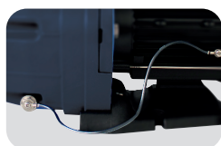
Bouchon de vidange inox pour raccorder la pompe à la terre
