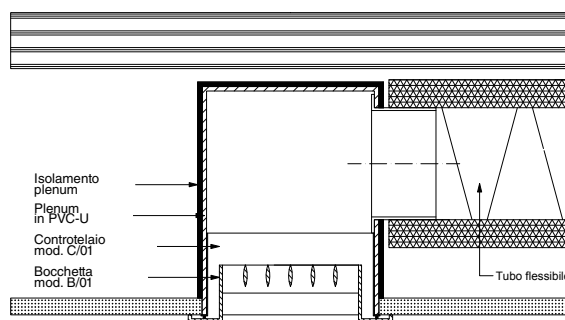
SEZIONE VISTA LATO CORTO
