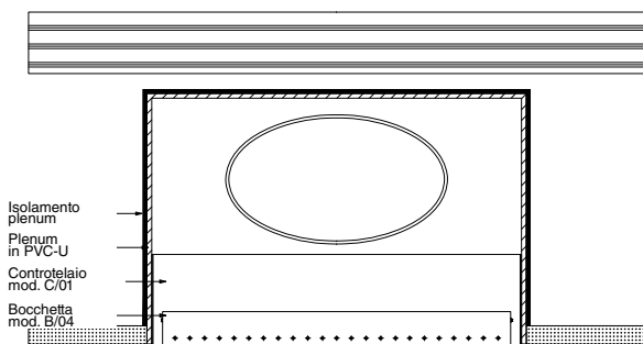
SEZIONE VISTA LATO LUNGO
