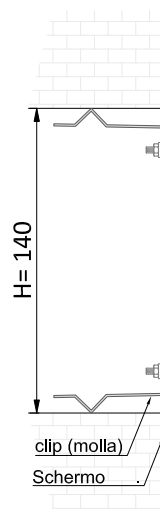
SEZIONE A-A
