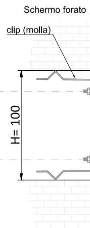
SEZIONE A-A
