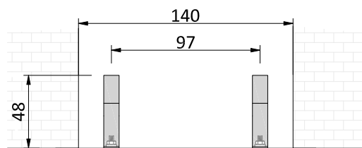
SEZIONE B-B
