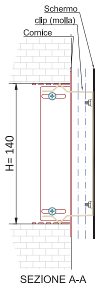
SEZIONE A-A
