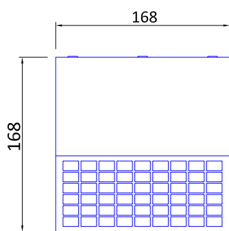
VISTA FRONTALE DELLA GRIGLIA (lato inf. con n. 54 fori quadri 15x15 mm)
