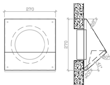
Disegno della griglia completa di base + coperchio (rimovibile) installati a muro
