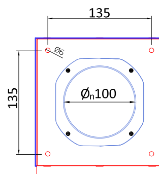
VISTA DEL RETRO DELLA GRIGLIA (spessore lamiera = 0.8 mm)
