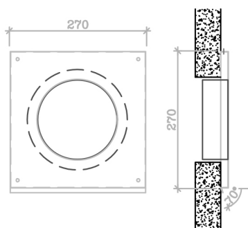
Disegno della "base" della griglia, dotata di gocciolatoio, fissata su parete esterna
