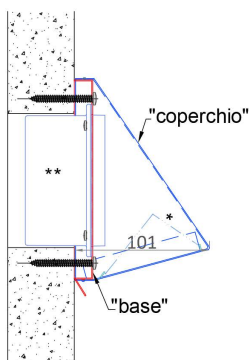
SEZIONE DELLA GRIGLIA CON FORO A MURO
