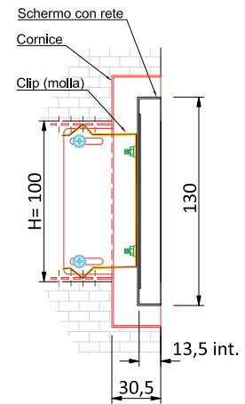
SEZIONE A-A
