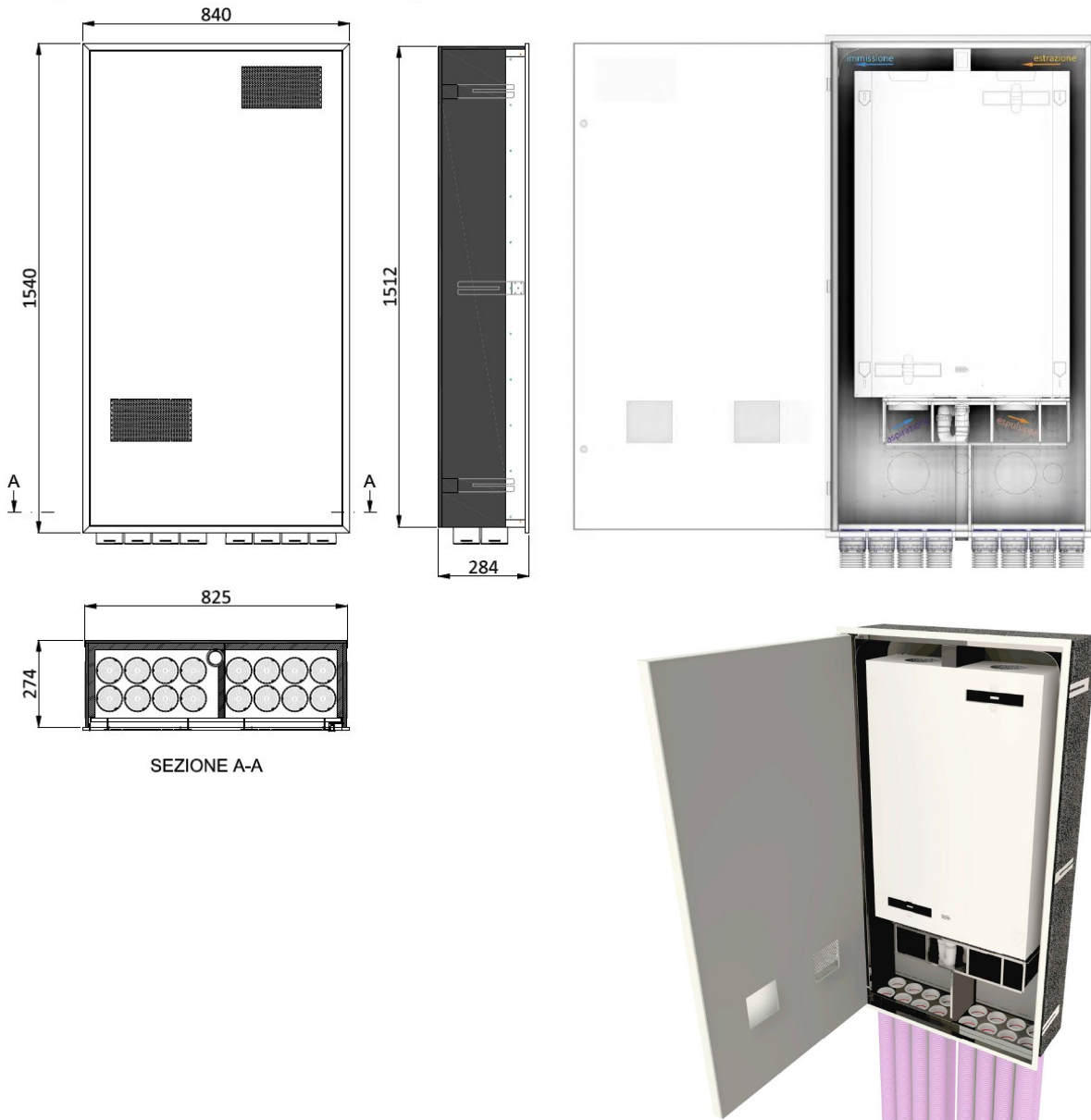
Disegno dimensionale del Silent Compact Box mod. VMSCB16X75B (misure in mm) - con unità SKY
